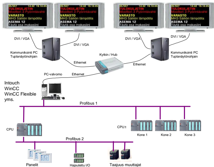
Esimerkki linjan / tehtaan prosessikaaviosta
